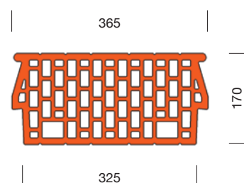
Porotherm 45/17 béléstest
