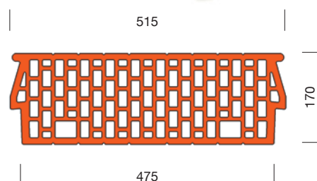
Porotherm 60/17 béléstest
